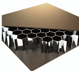
LAH Anima interna Nido d'ape in alluminio
